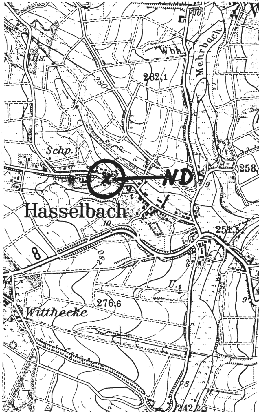
Ausschnittvergrößerung 1:10 000 aus der Top. Karte 1:2 Blatt Nr. 5511 Bendorf, Herstellung der Druckunterlagen Landesvermessungsamt Rheinland-Pfalz, 1982
