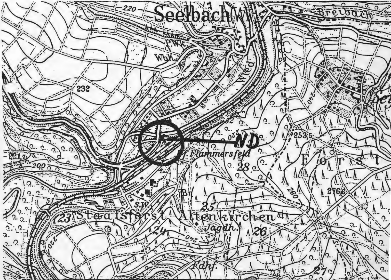
Ausschnittvergrößerung 1:10 000 aus der Top.Karte 1:25 000, Bl.-Nr. 5314 Altenkirchen
